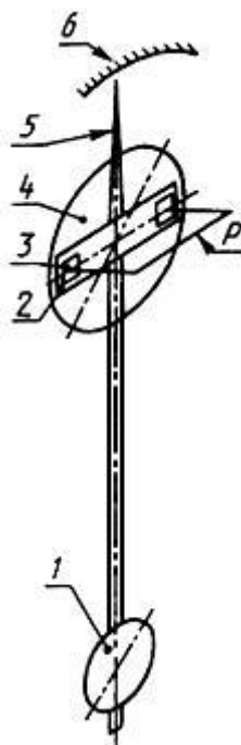
1 - маятник; 2 - держатель образцов; 3 - образец; 4 - металлическое контртело; 5 - стрелка; 6 - шкала момента трения
